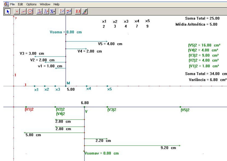
Figura 3: La varianza como una media
