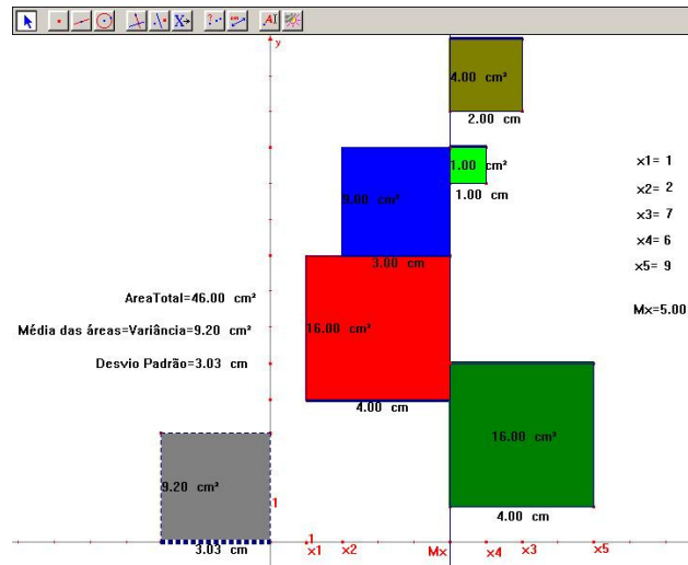
Figura 2: Representación gráfica de la varianza
