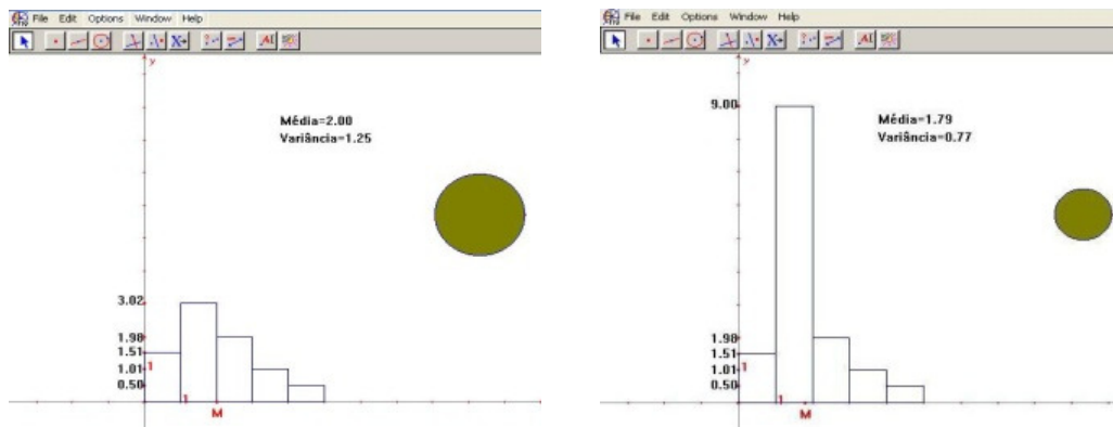
Figure 1: Varianza y frecuencia
