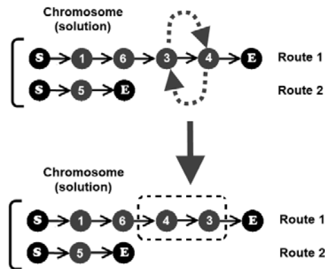
Figura 4: O processo de mutação.
