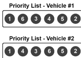
Figura 1: Listas prioritárias para dois veículos numa instância com seis vértices.
